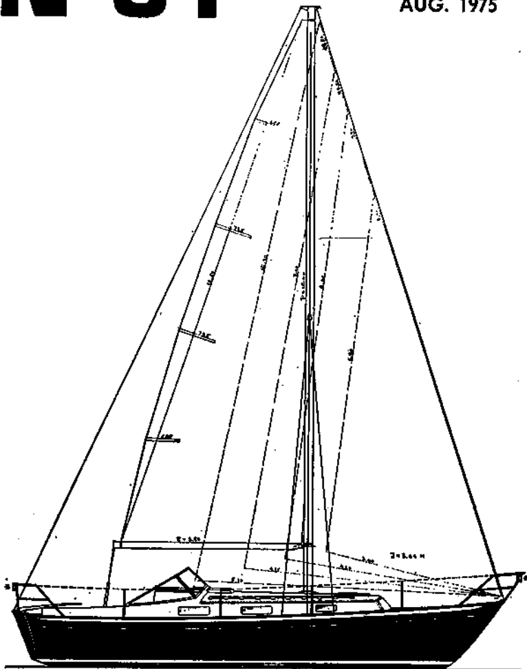
Masstab 1:100.
