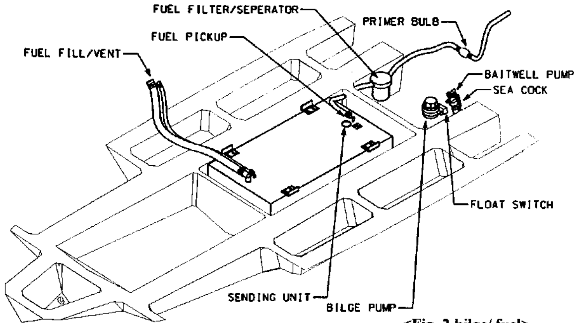
<Fig. 2 bilge/ fuel>
