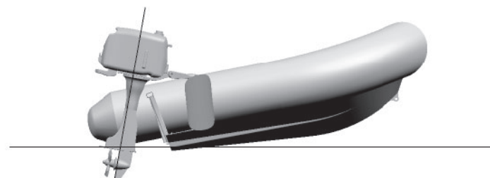
L'avant du bateau déjauge, trop de trim positif
