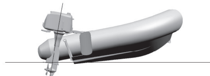
Bug oben, zu viel Trimm nach außen
